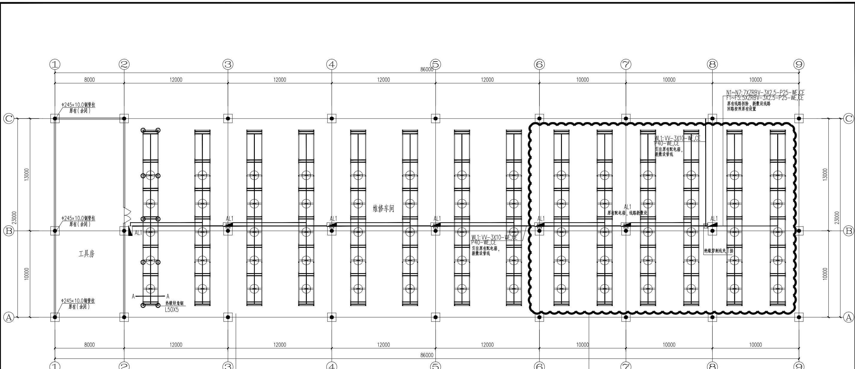
首层改造电气平面图 1:150
