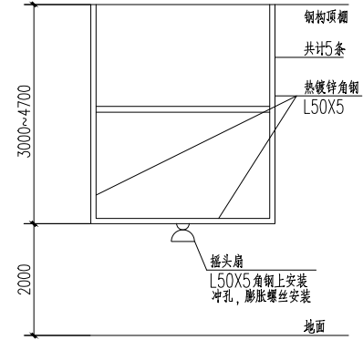
风扇及灯具支架大样图A-A 1:150
